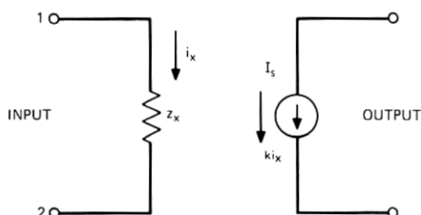
Fig. 1—Basic amplifier.
